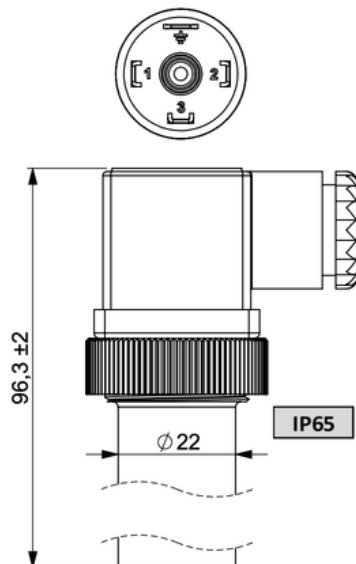
EN 175 301-803-A
