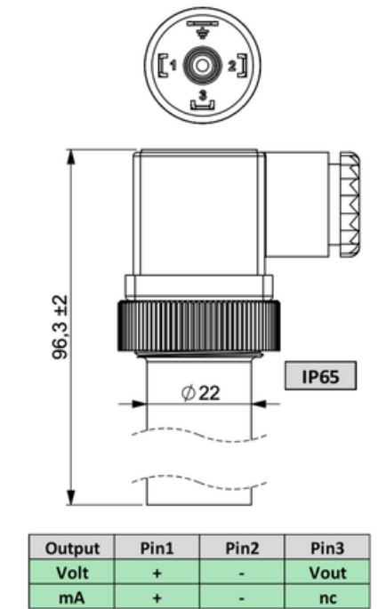
EN 175 301-803-A
